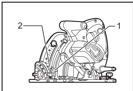
► 1. Vis de serrage 2. Butée de limite inférieure de la lame
