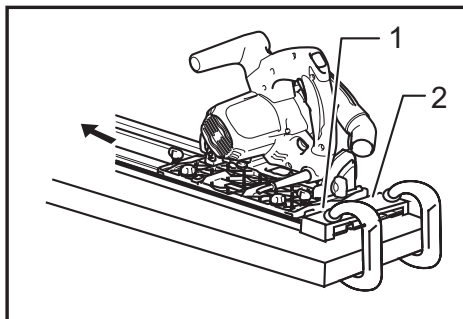
► 1. Borde trasero de base de la herramienta 2. Tope fijo
