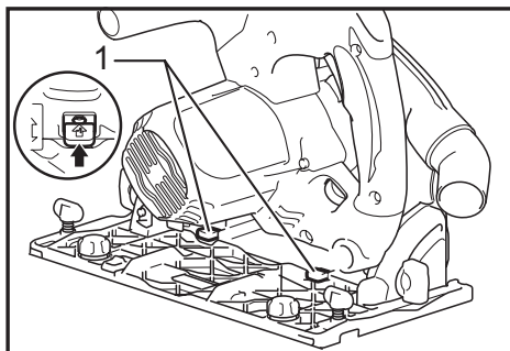
► 1. Levier de changement d'angle de coupe en biseau
