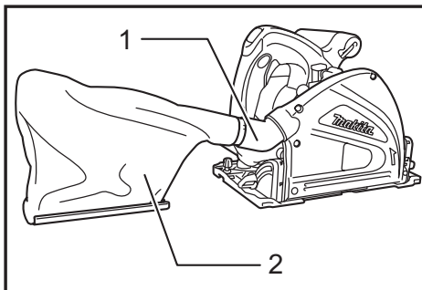
► 1. Dust port 2. Dust bag
